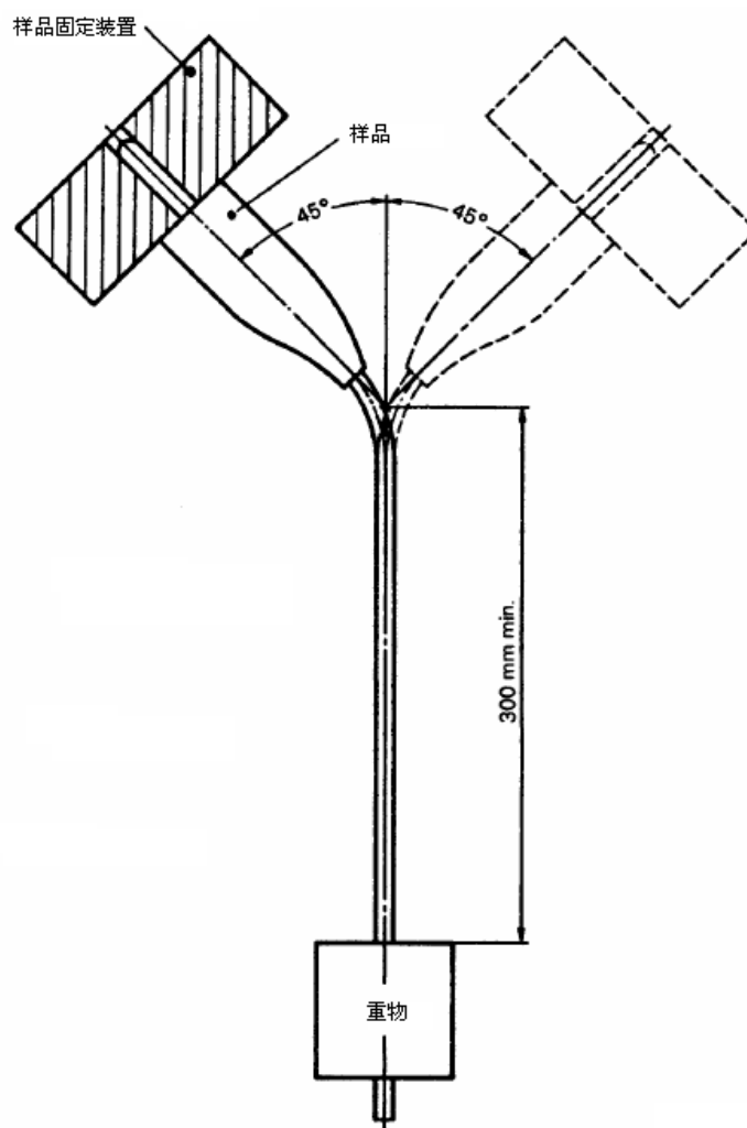
图10 弯曲试验装置
