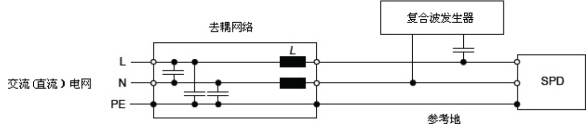
图1 用于单相电源去耦网络的示例
