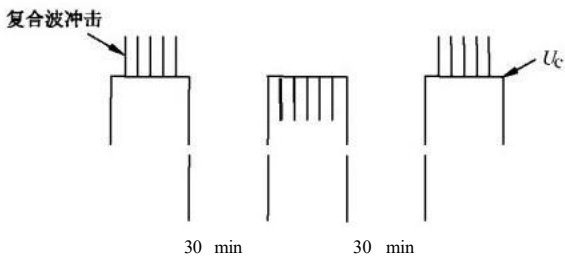
图 10 III类试验的动作负载试验时序图
