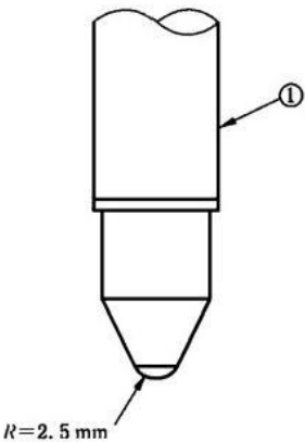
图19 球压试验装置
