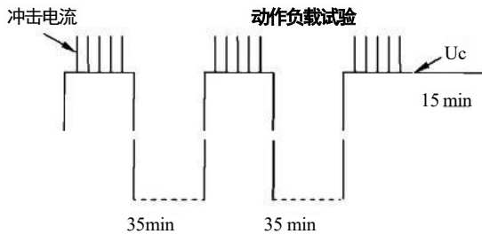
图8 I 类、II 类试验的动作负载时序图
