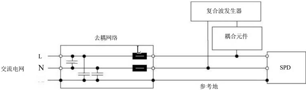
图 2 用于单相电源去耦网络的示例
