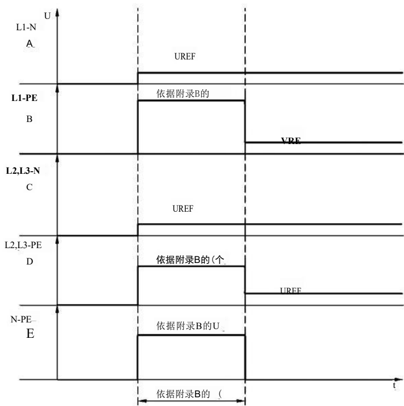
图16 在高(中)压系统故障引起的TOV 下用于 TT 系统的SPD 端子上预期电压的相应时序图
