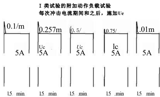
图 9 I 类试验的附加动作负载试验时序图
