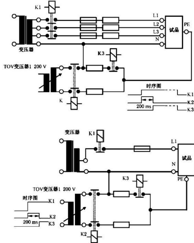
图 H.1 用于高(中)压系统故障引起 TOV 下用于 TT 系统 SPD 试验的三相和单相电路的示例
