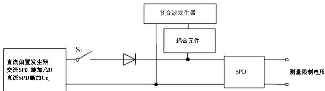
图 4 测量限制电压的替代试验
