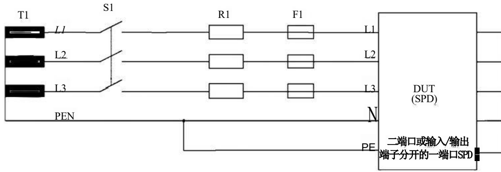
b) 负载侧所有端子短路的测试
