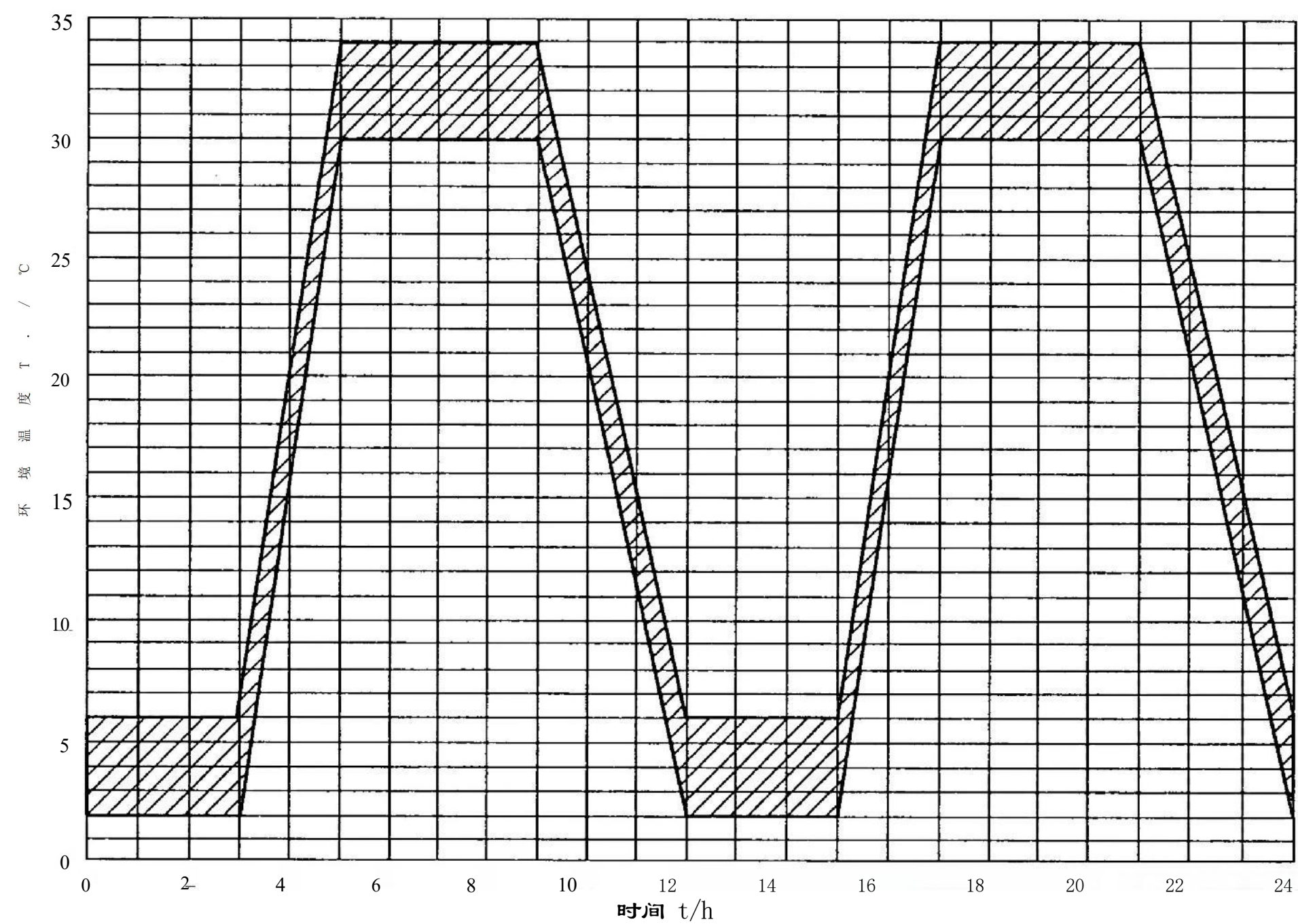
图 1 4 环境循环试验方案 A,RH≥90%
