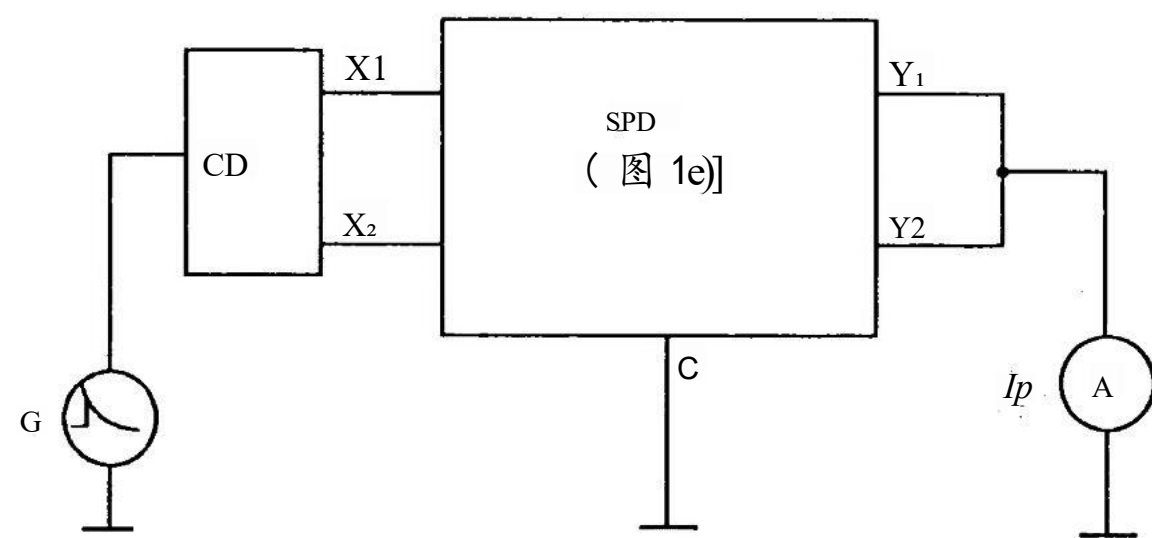
图 E.5 共模最大允通电流的测定
