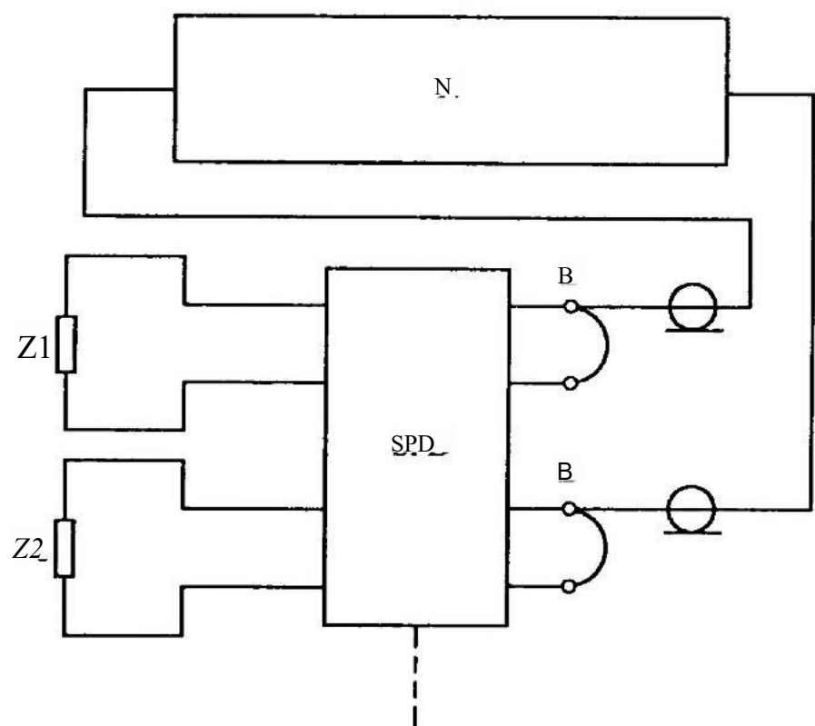
图 1 1 检验误码率的试验电路
