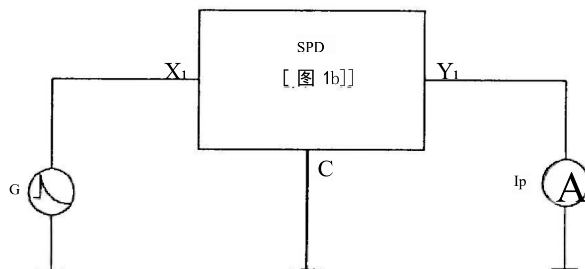
图 E.1 差模允通电流的测定
