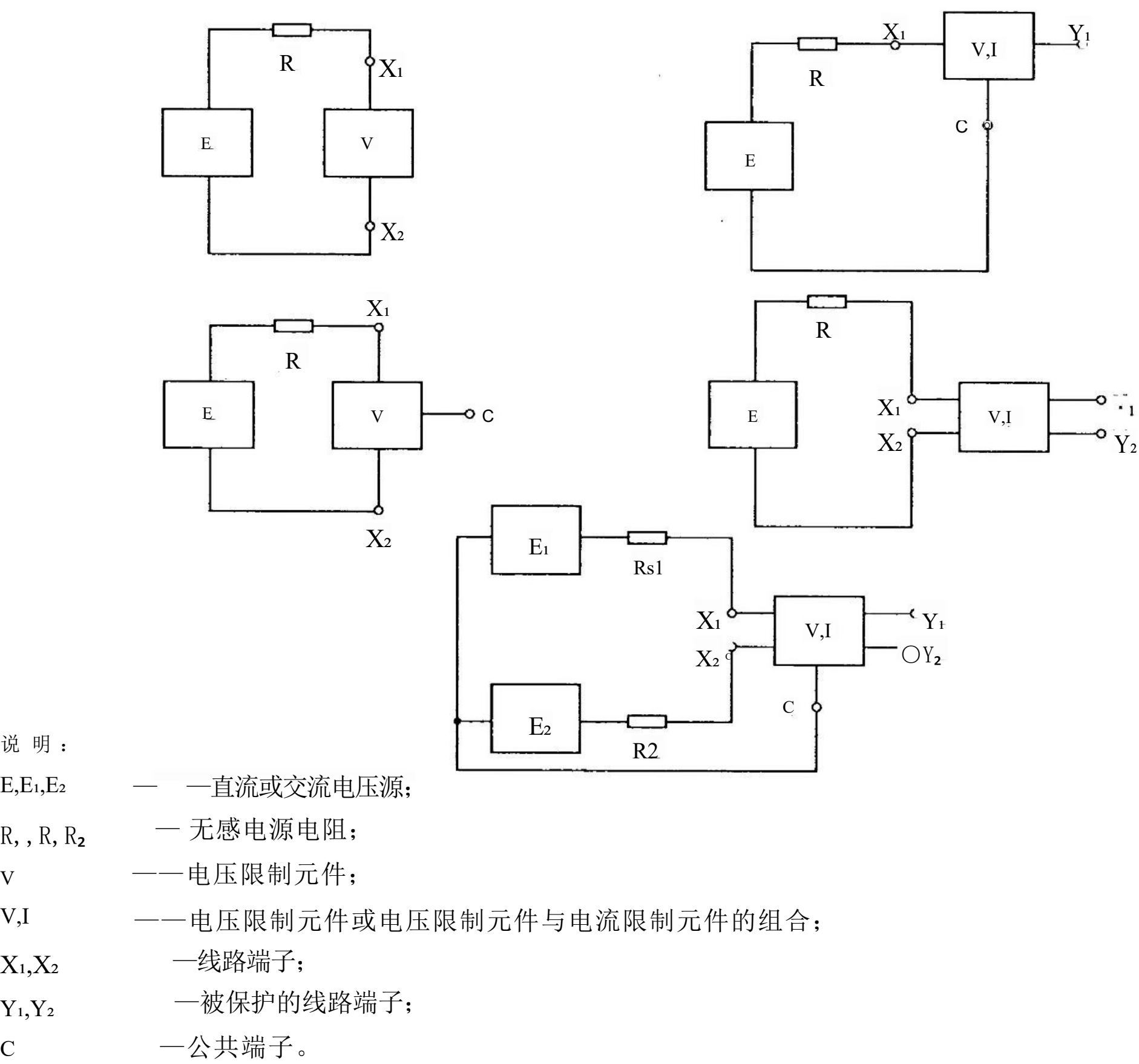
图 1 3 高温/高湿度耐受试验和环境循环试验电路
