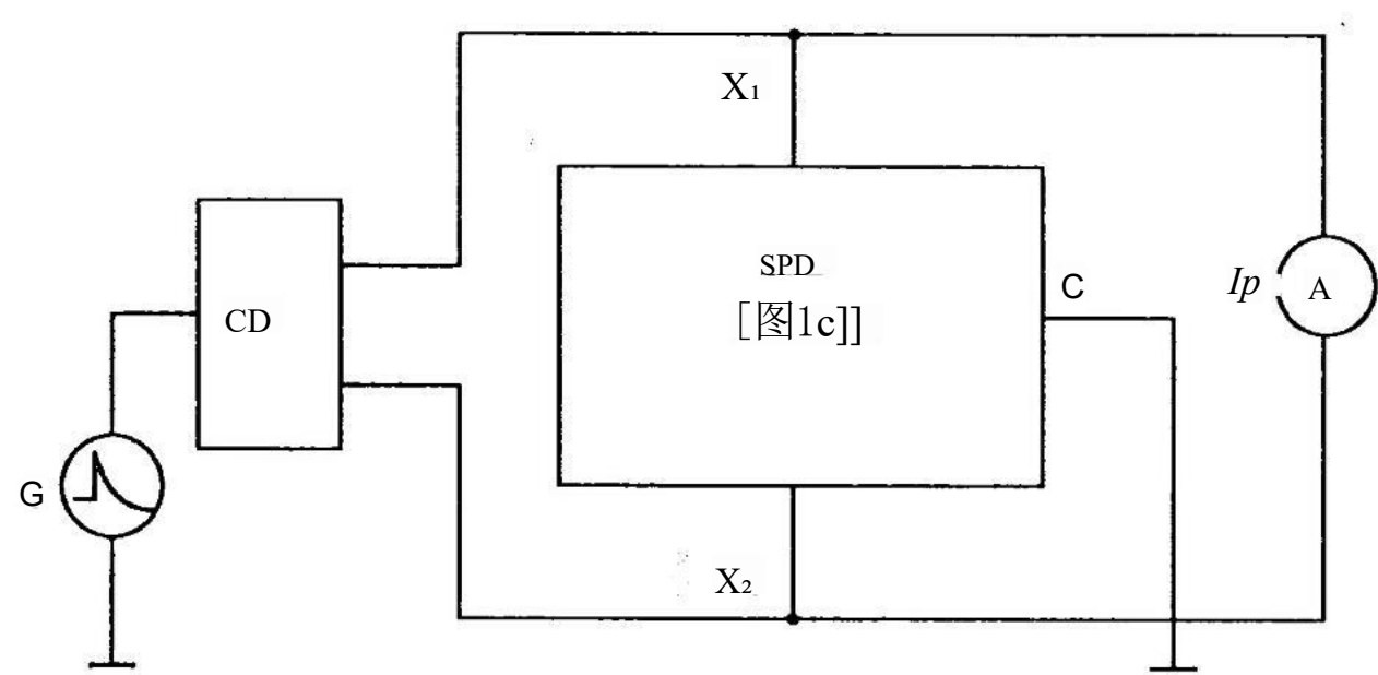
图 E.3 差模允通电流的测定
