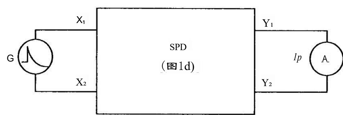
图 E.4 差模允通电流的测定
